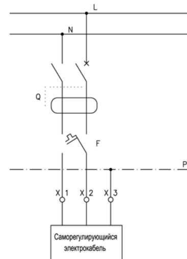
Рис. 5. Схема подключения электрообогрева кровельной воронки HL62.1BH к электрической сети.
