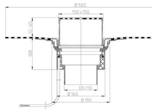
Рис. 2. Кровельная воронка HL62.1BH/1.
