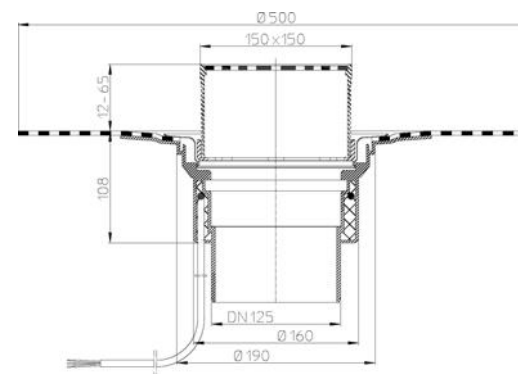
Рис. 3. Кровельная воронка HL62.1BH/2.
