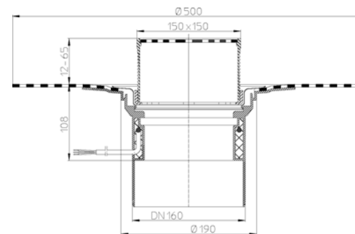
Рис. 4. Кровельная воронка HL62.1BH/5.
