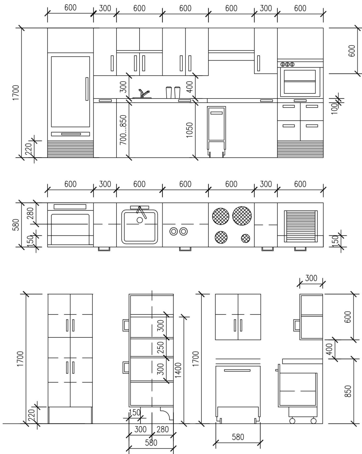
Рис. 18 – Обладнання кухні
