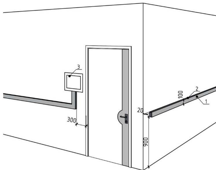
Рис.39 Приклад улаштування тактильних інформаційних позначок при- міщень при неможливості розміщення тактильної таблички справа від дверей: 1-інформаційна направляюча, 2- тактильна інформаційна позначка, 3- інфор- маційна тактильні табличка, що дублює текстову інформацію у тактильному вигляді плоско дру- кованого тексту та шрифтом Брайля
