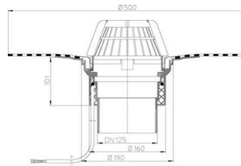
Рис. 3. Кровельная воронка HL62.1H/2.
