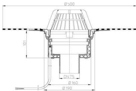
Рис. 1. Кровельная воронка HL62.1H/7.
