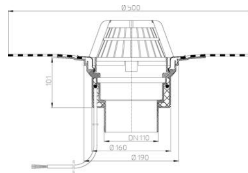
Рис. 2. Кровельная воронка HL62.1H/1.
