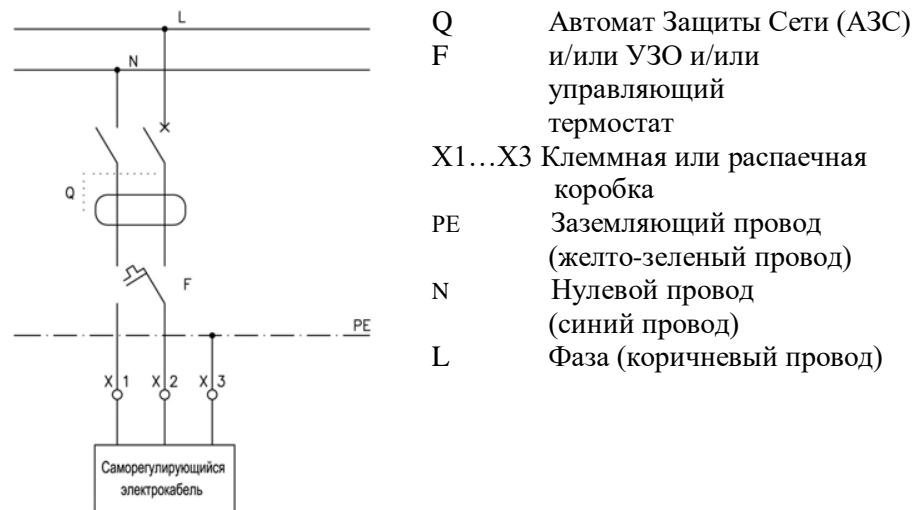
Рис. 5. Схема подключения электрообогрева кровельной воронки HL62.1H к электрической сети.
