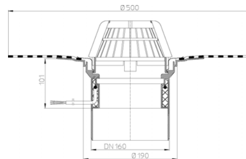
Рис. 4. Кровельная воронка HL62.1H/5.
